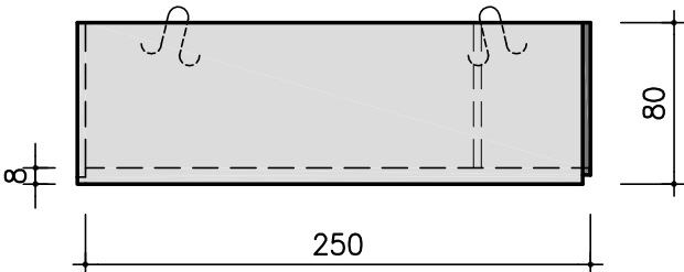
VISTA LATERALE Scala 1:50
